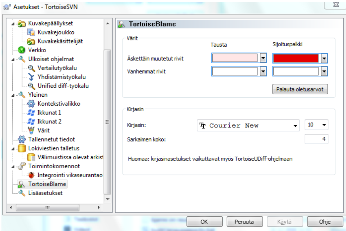
Kuva 4.92. Asetusikkuna, TortoiseBlame-sivu
