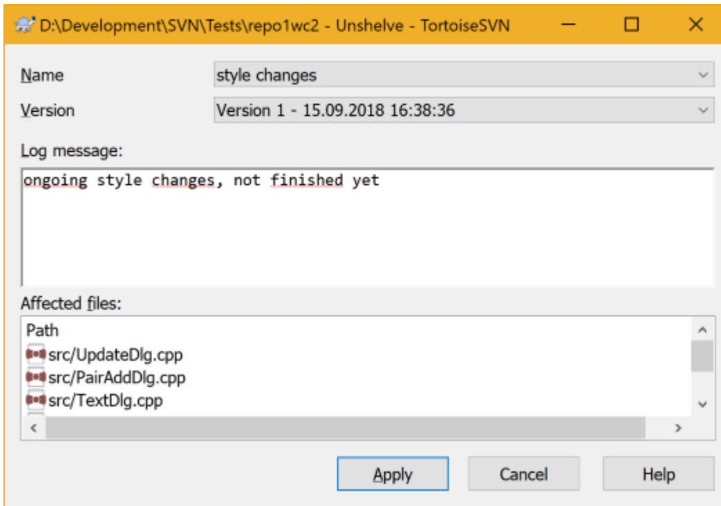
Kuva 4.17. Unshelve dialog
