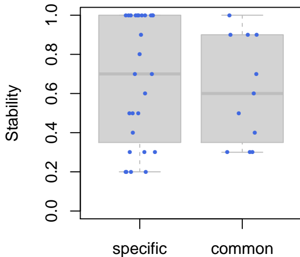
Dataset: expO.colon.ras
