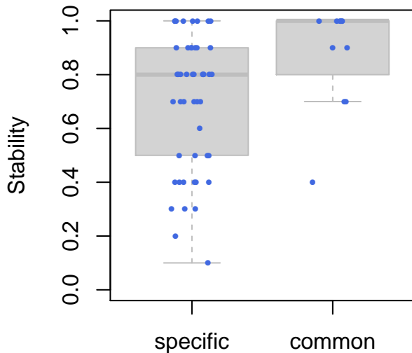
Dataset: jorissen.colon.ras
