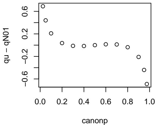
U(0,1)
