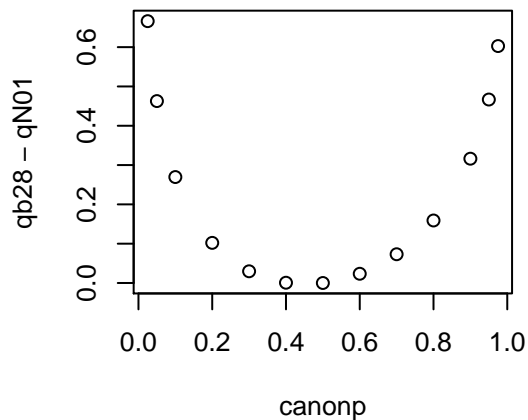
Beta(2,8)
