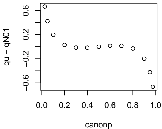
U(0,1)
