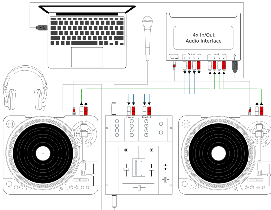
Figure 1: Mixxx gemeinsam mit Plattenspielern und externen Mixer verwenden
