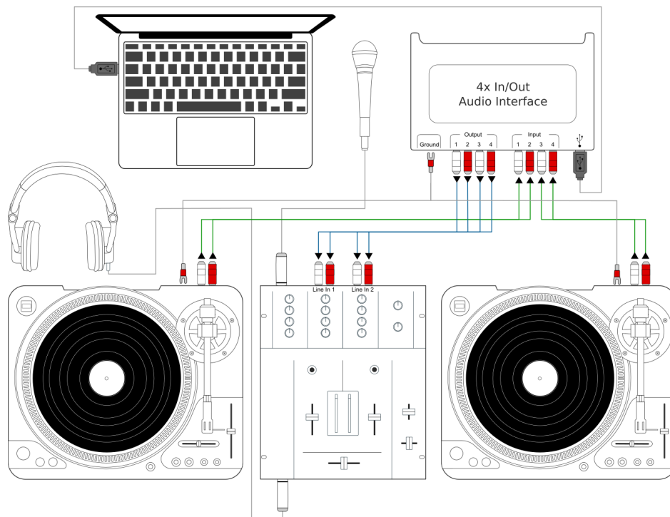
Figure5: Mixxx gemeinsam mit Plattenspielern und externen Mixer verwenden
