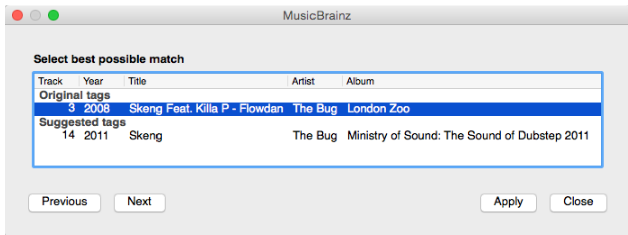
Figure4: Mixxx-Bibliothek - MusicBrainz-Assistent
