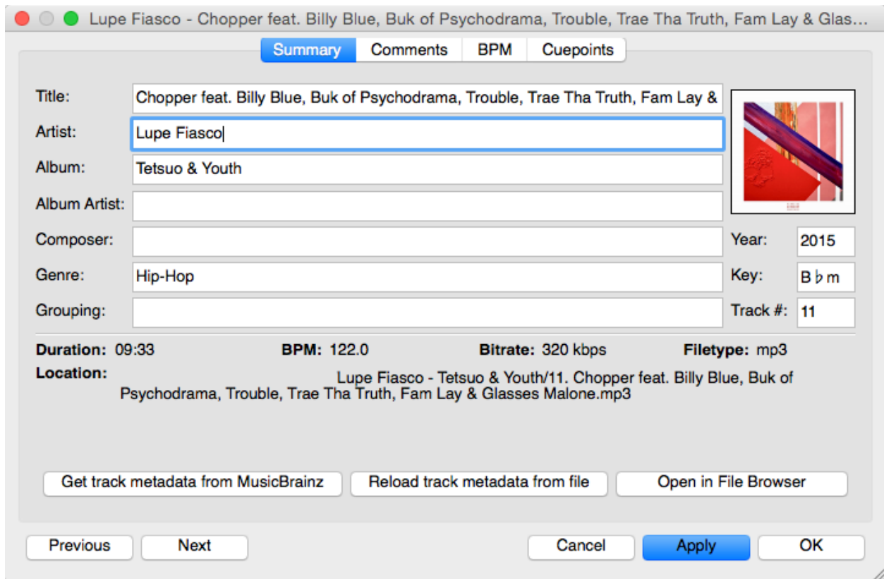
Figure3: Mixxx-Bibliothek - Eigenschaften-Editor
